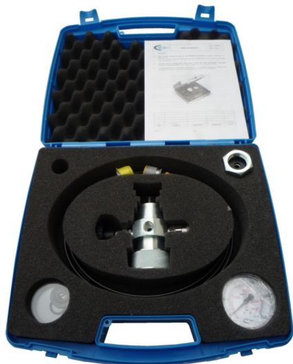
Внешний вид комплекта PCM250M8
