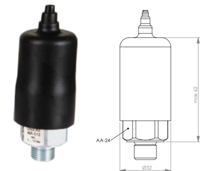
Внешний вид реле давления серия DS3 с исполнением контактов FAC, NA, NC
